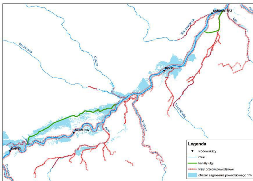
Rysunek 7 Lokalizacja kanałów ulgi (kanal ulgi Strumień i kanal ulgi Trześniówka)
