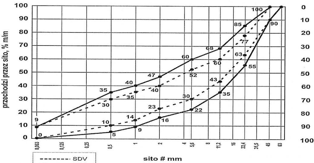
Rys. 12. Uziarnienie mieszanki niezwiązanej 0/45 dla podbudowy zasadniczej
